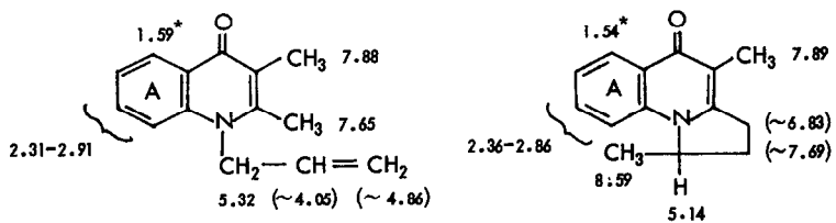
Fig. 1. N.m.r. Spectral Data a,b (chemical shift : \tau )
